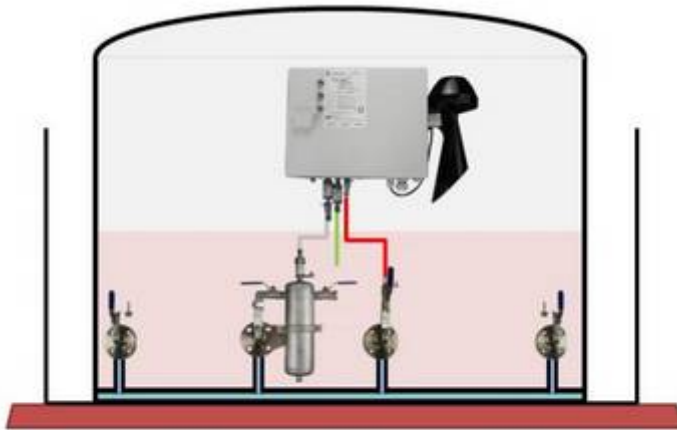
VLX 330/Ex am Tank nach DIN 4119
