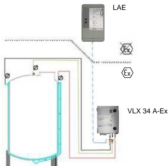
VLX .. A-Ex avec LAE au niveau du réservoir selon DIN 6618/2
