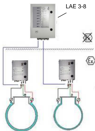
VLX 330 A-Ex avec LAE 3-8 sur plusieurs réservoirs selon DIN 6608/2
