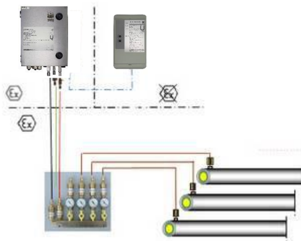
VLX 330 A-Ex pour surveiller les conduites
